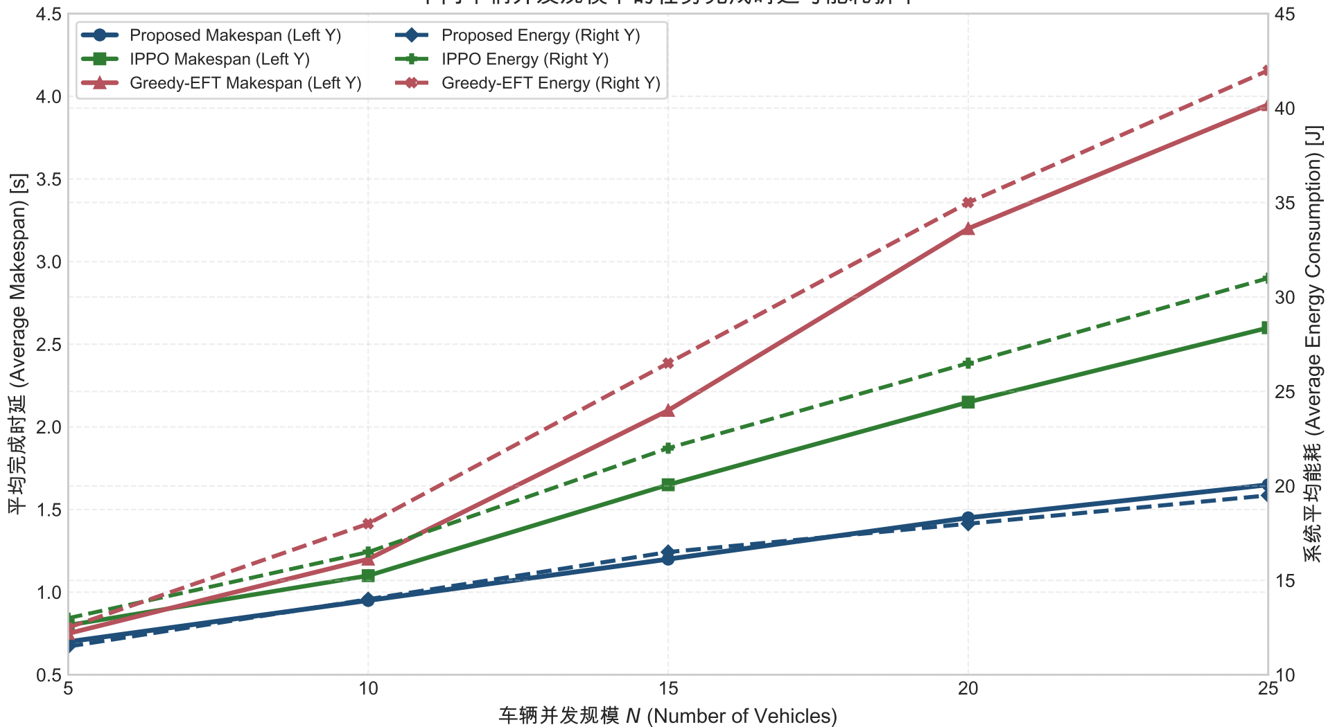
不同车辆并发规模下的任务完成时延与能耗折中
