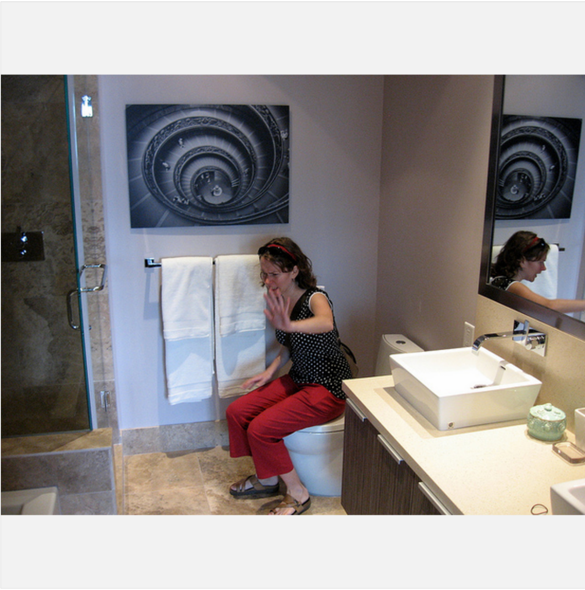
GQA
