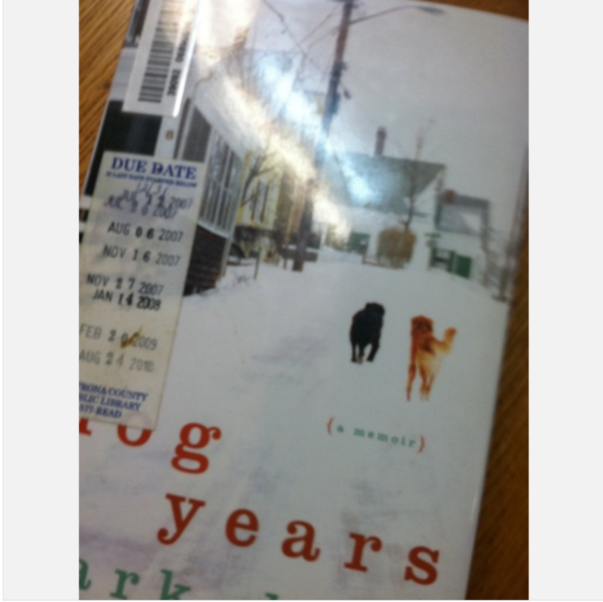
VizWiz
