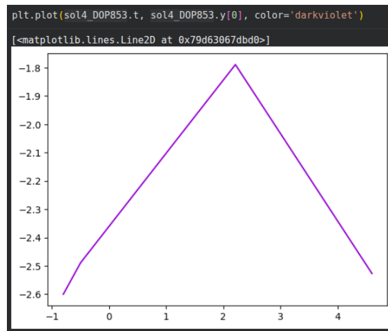
Figura 4: Captura de pantalla de la gráfica resultante de sol4 calculado con DOP853
