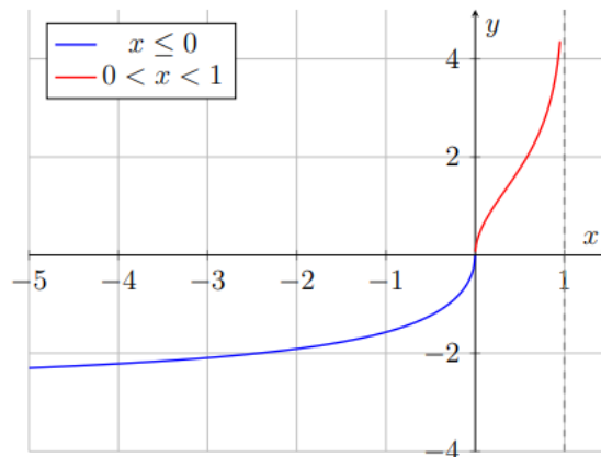
Figura 6: Gráfica de la función por partes con C = 0
