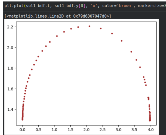
Figura 1: Captura de pantalla de la gráfica resultante de \text{sol1} calculado con BDF
