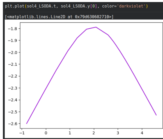
Figura 3: Captura de pantalla de la gráfica resultante de sol4 calculado con LSODA
