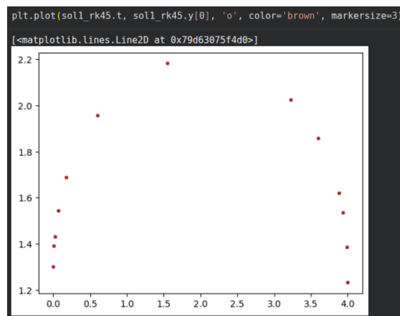
Figura 2: Captura de pantalla de la gráfica resultante de \text{sol1} calculado con RK45
