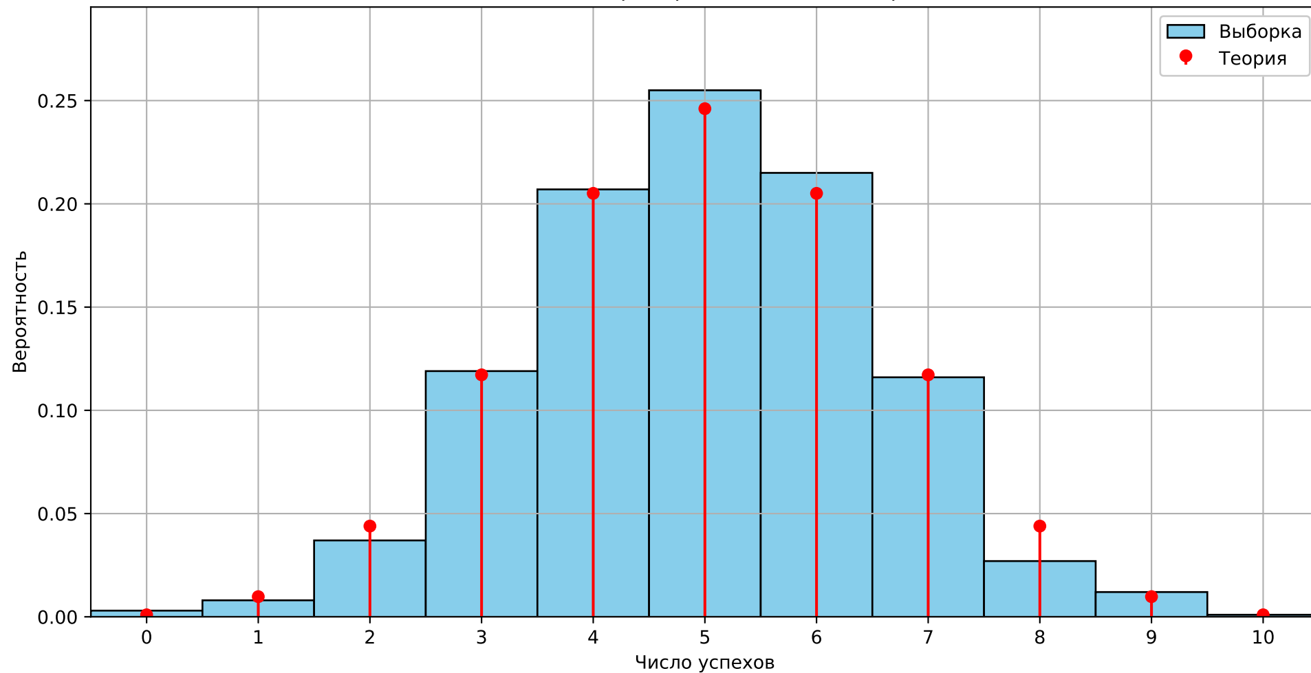
Биномиальное распределение ( n=10 , p=0.5 )
