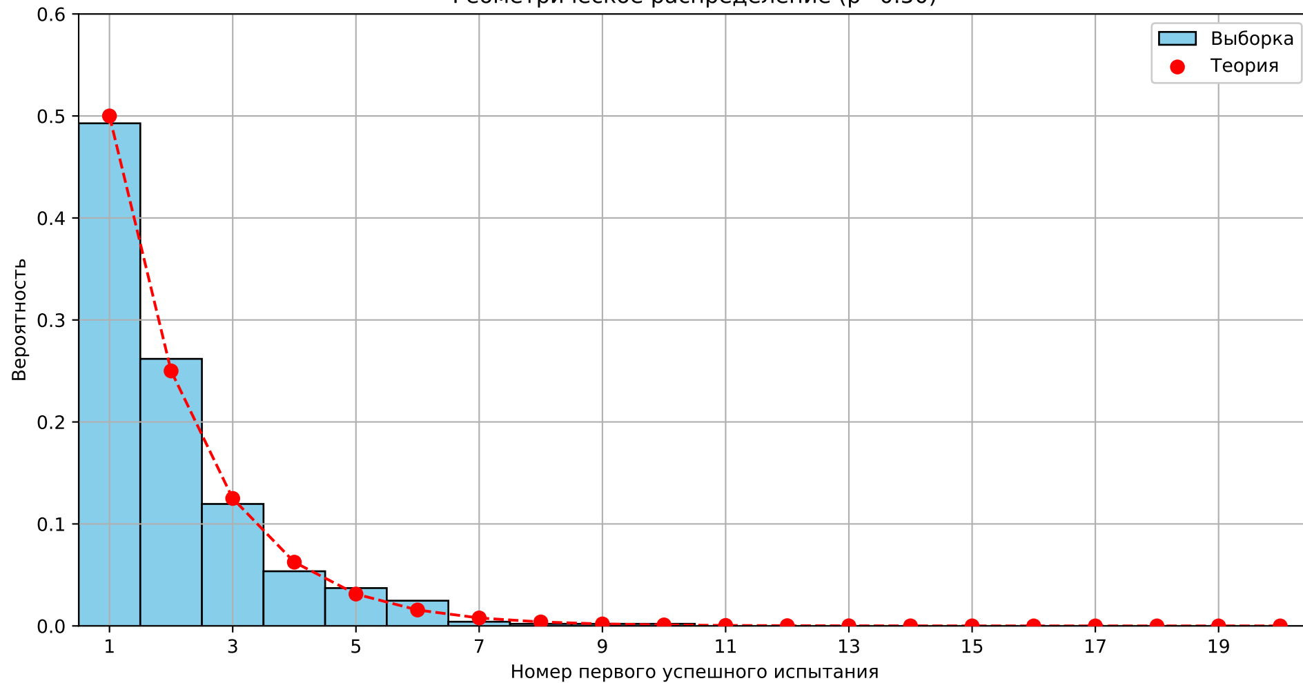
Геометрическое распределение ( p=0.50 )
