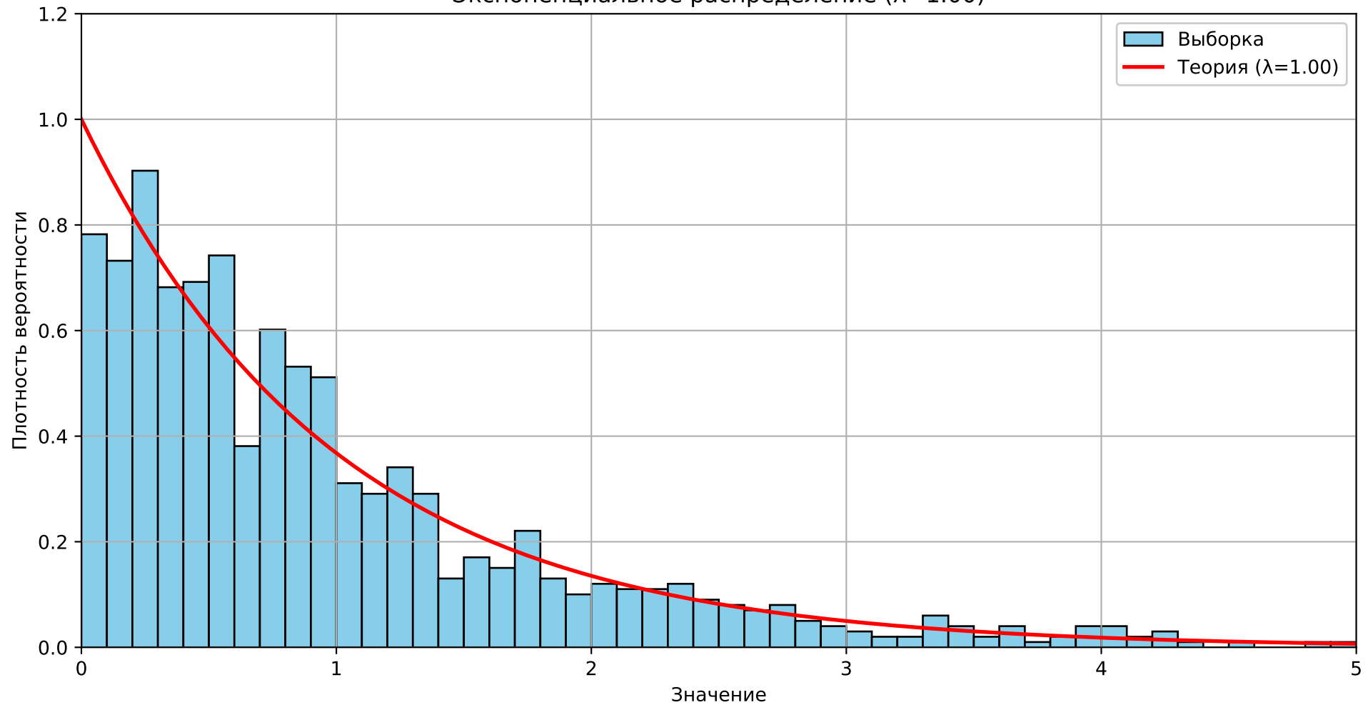
Экспоненциальное распределение ( \lambda=1.00 )
