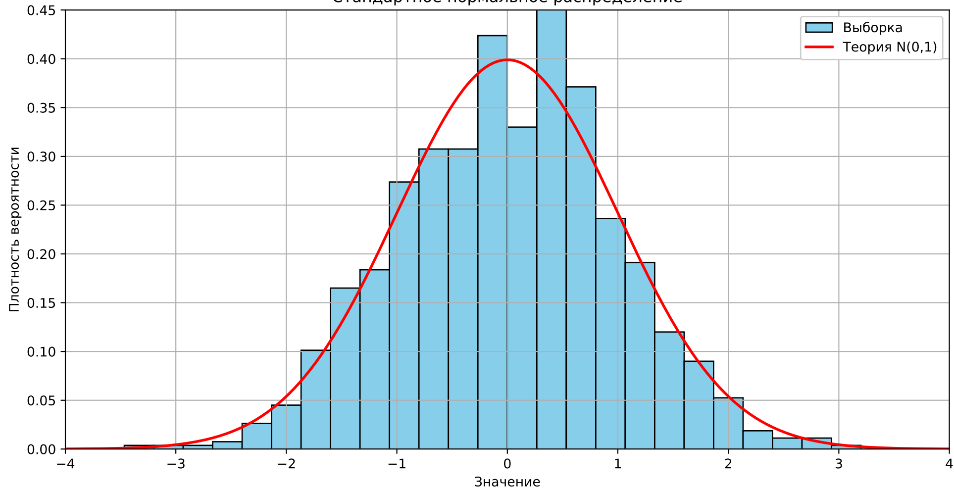
Стандартное нормальное распределение
