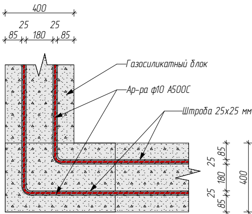
Узел 1. Армирование угла кладки
