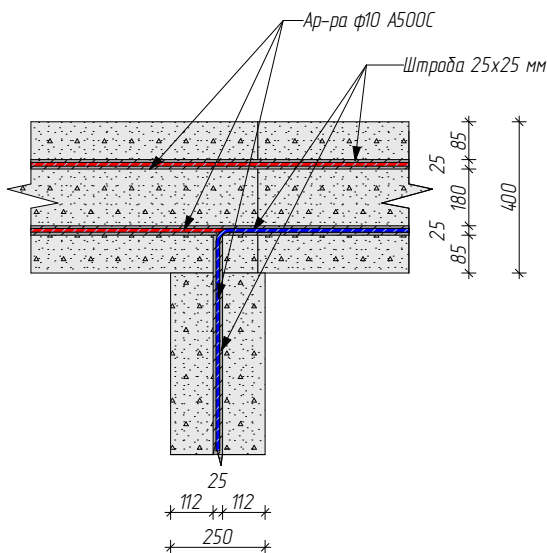
Узел 2. Армирование кладки блоков 250 мм
