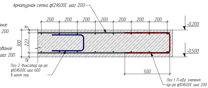
Сечение по фундаментной плите
