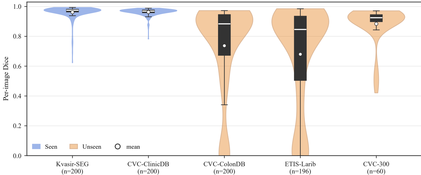
Per-image Dice distribution per dataset (WaveLite-DG)
