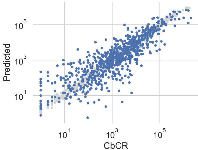
Var: ln_emp R2: 0.72
