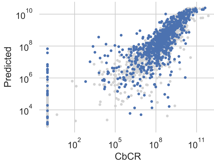
Var: ln_t_at R2: 0.53
