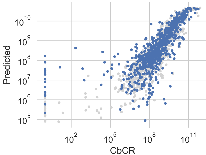
Var: ln_revt R2: 0.47
