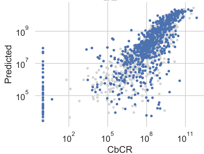
Var: ln_t_at R2: 0.50
