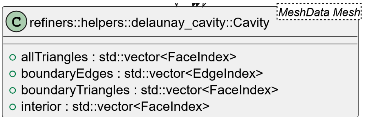
Figura 35: Representación UML de la estructura Cavity
