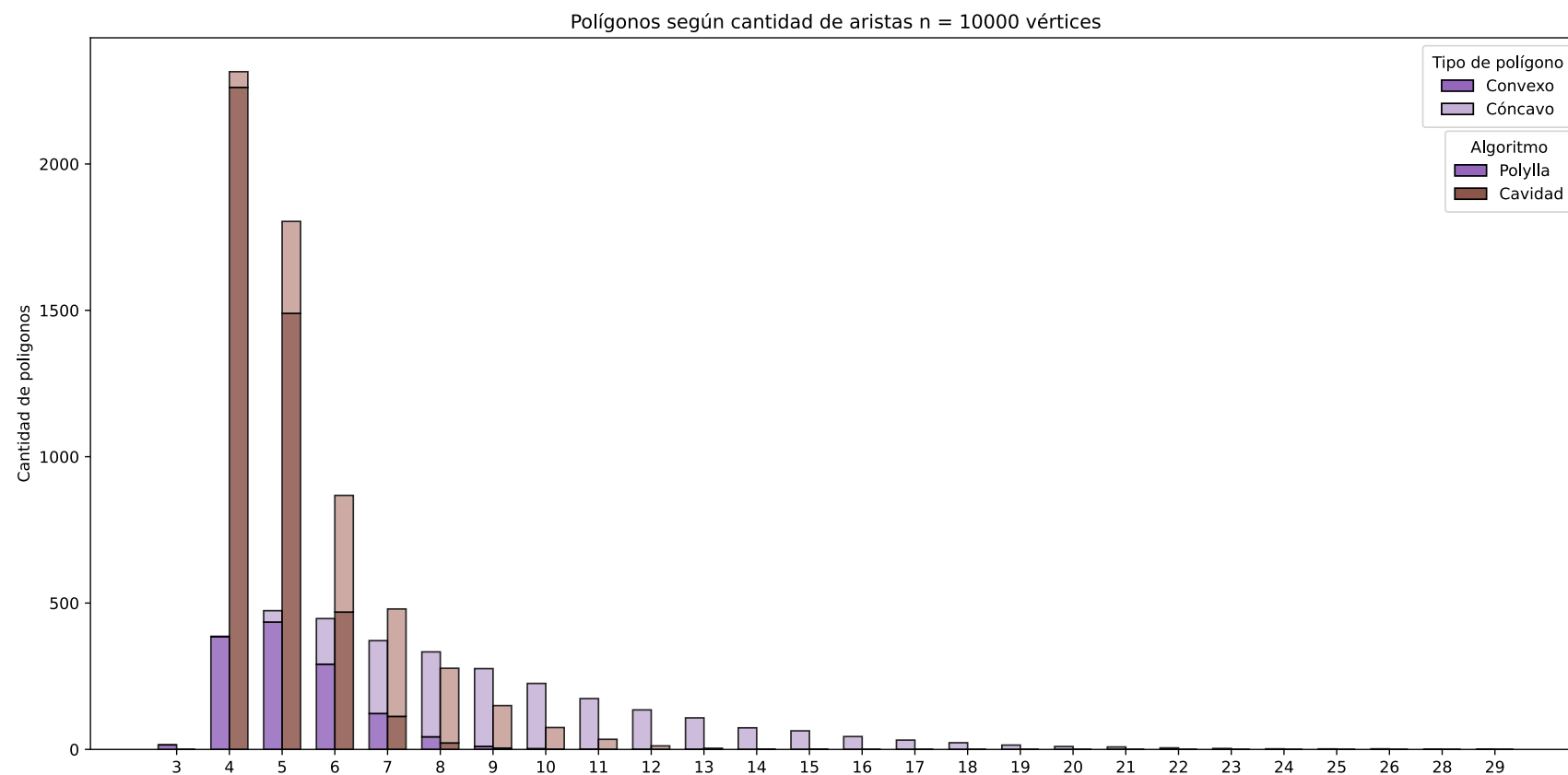
Figura 52: Distribución promedio de polígonos según cantidad de aristas con 10000 vértices
