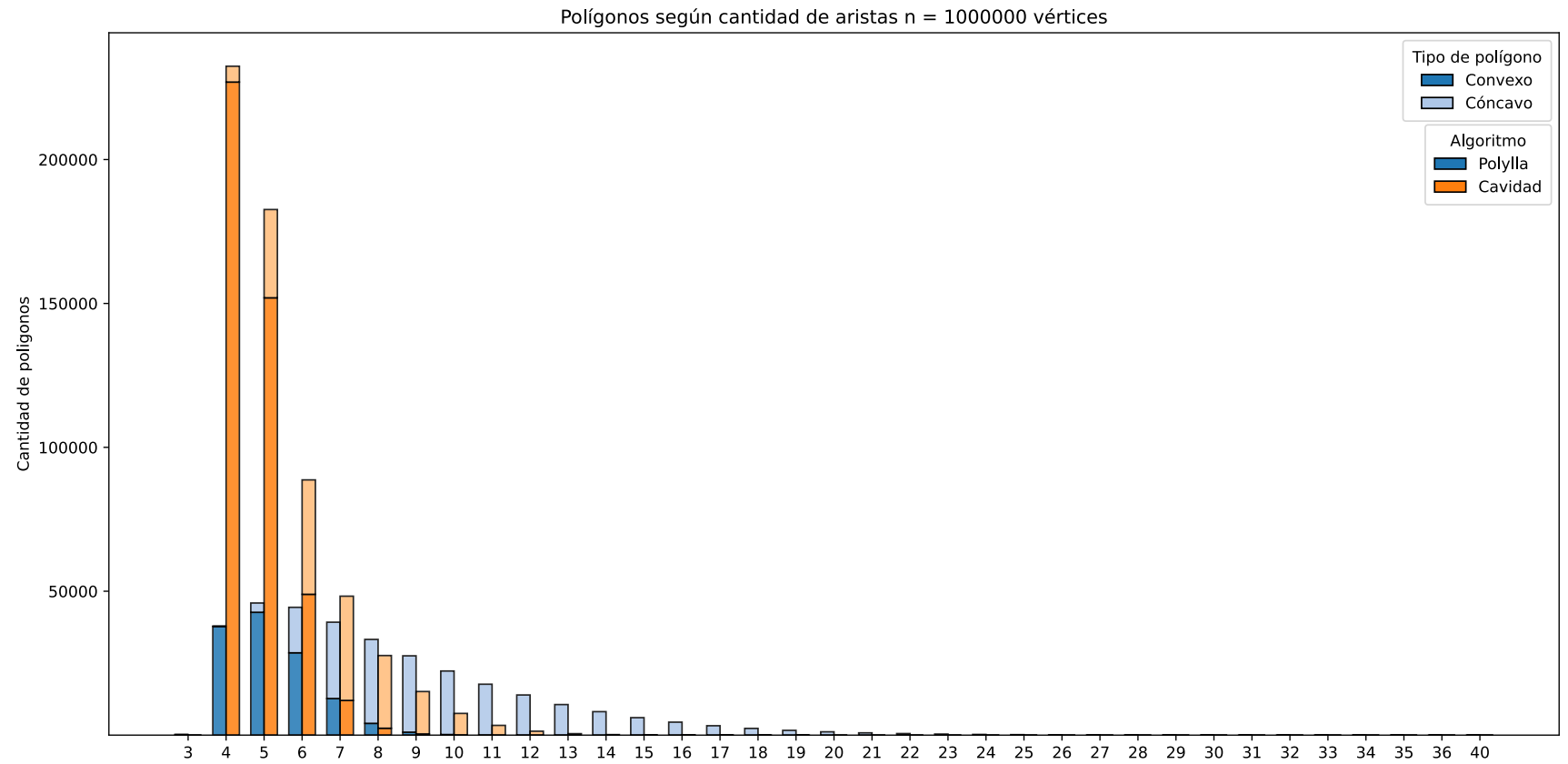
Figura 54: Distribución promedio de polígonos según cantidad de aristas con 1000000 de vértices
