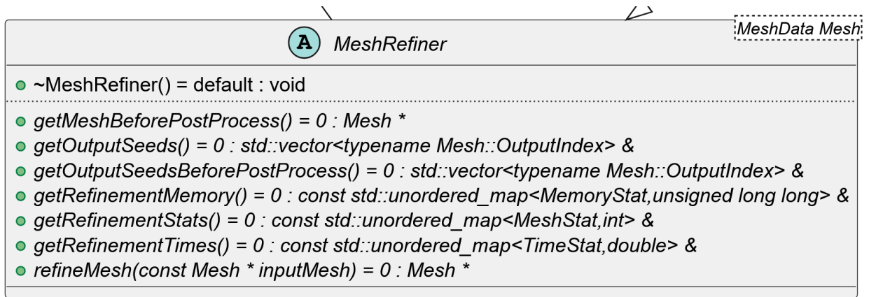
Figura 28: Representación UML de la clase MeshRefiner
