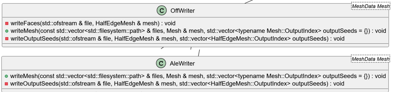
Figura 27: Representación UML de las clases OffWriter y AleWriter
