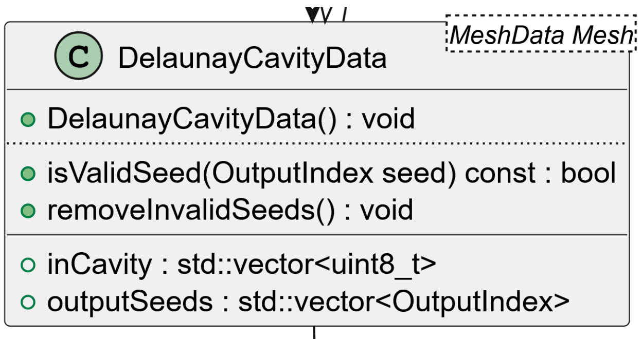
Figura 36: Representación UML de la clase DelaunayCavityData
