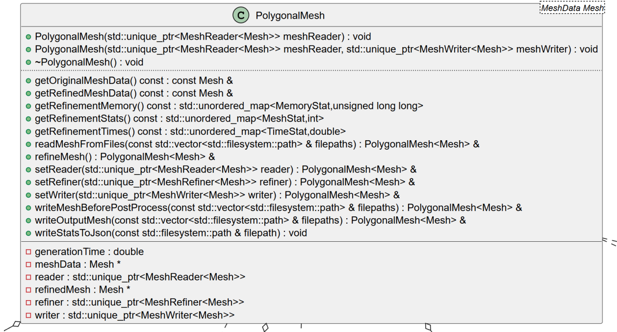
Figura 21: Representación UML de la clase PolygonalMesh
