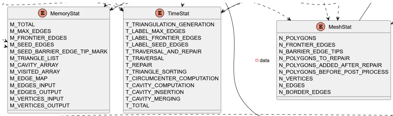
Figura 31: Representación UML de enumeraciones para estadísticas
