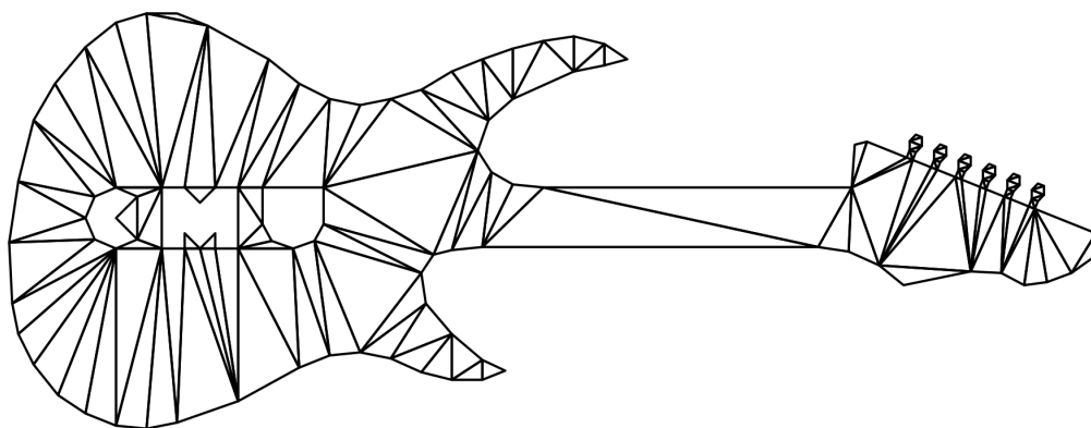
Figura 13: Triangulación restringida del PSLG de la Figura 10 con triángulos extra removidos [6]
