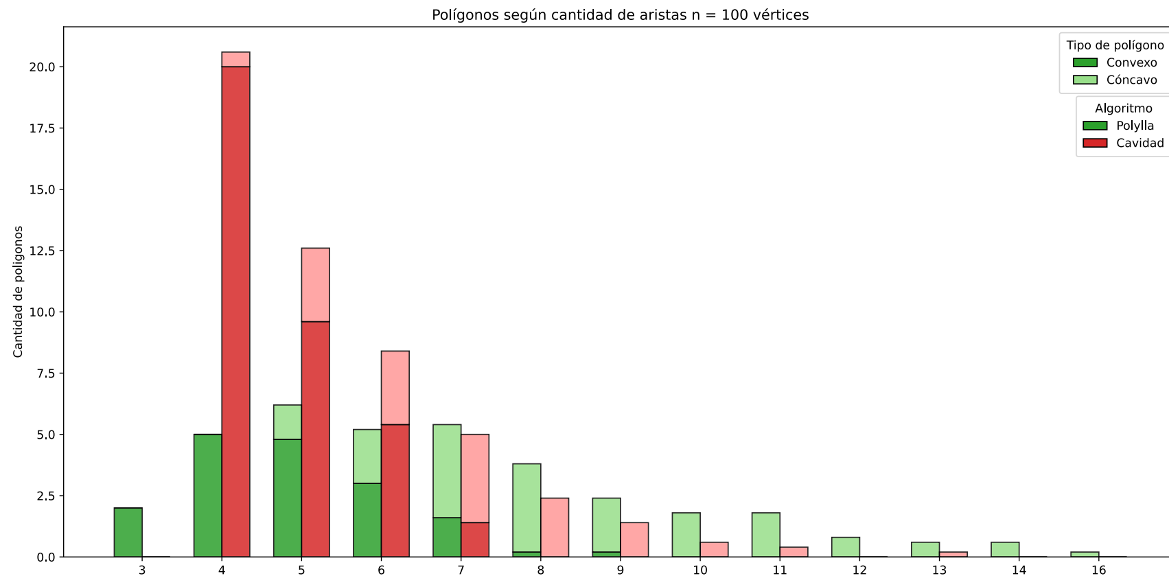
Figura 50: Distribución promedio de polígonos según cantidad de aristas con 100 vértices
