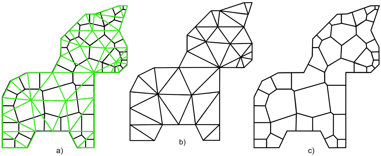
Figura 5: a) Triangulación de Delaunay y Diagrama de Voronoi superpuesto, b) Triangulación de Delaunay restringida, c) Diagrama de Voronoi restringido [3]
