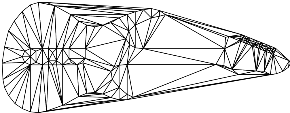
Figura 12: Triangulación restringida del PSLG de la Figura 10 [6]
