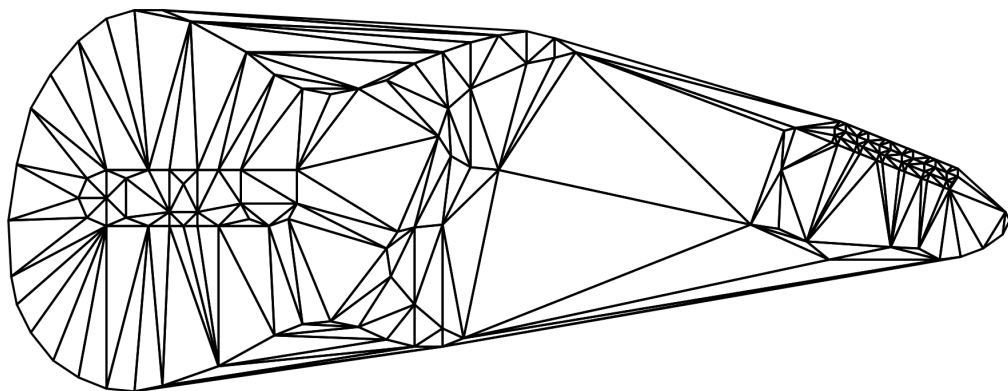
Figura 11: Triangulación de la cerradura convexa del PSLG de la Figura 10 con segmentos originales faltantes [6]
