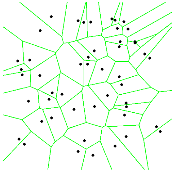
Figura 4: Ejemplo de diagrama de Voronoi. Fuente: Software Detri2[2]
