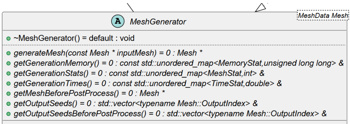
Figura 31: Representación UML de la clase MeshGenerator
