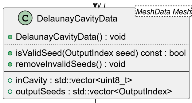
Figura 39: Representación UML de la clase DelaunayCavityData
