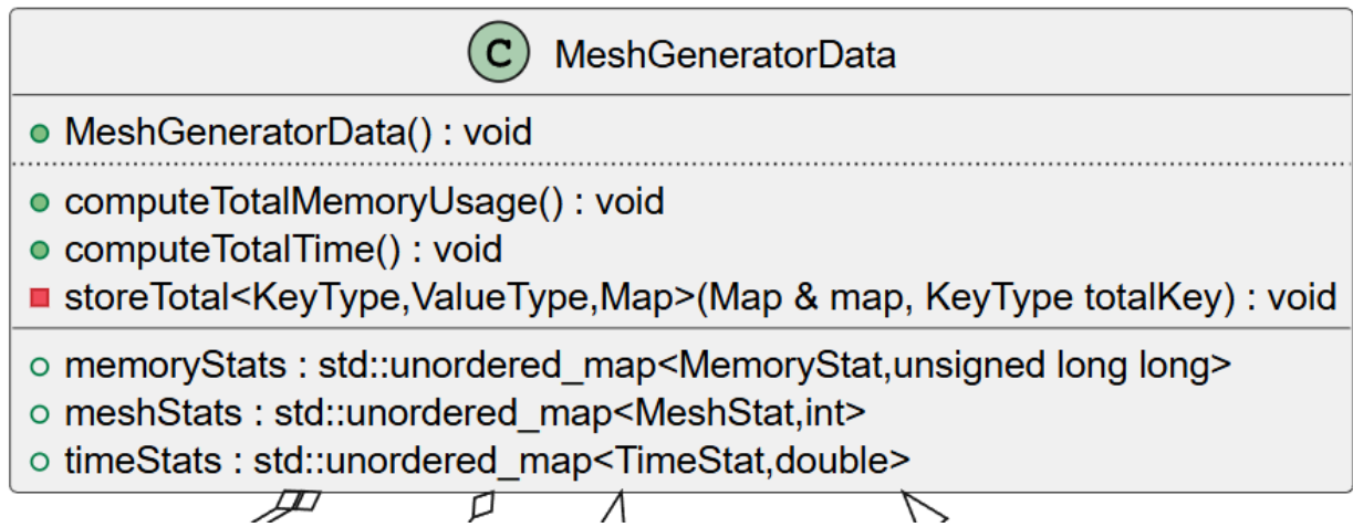
Figura 33: Representación UML de la clase MeshGeneratorData
