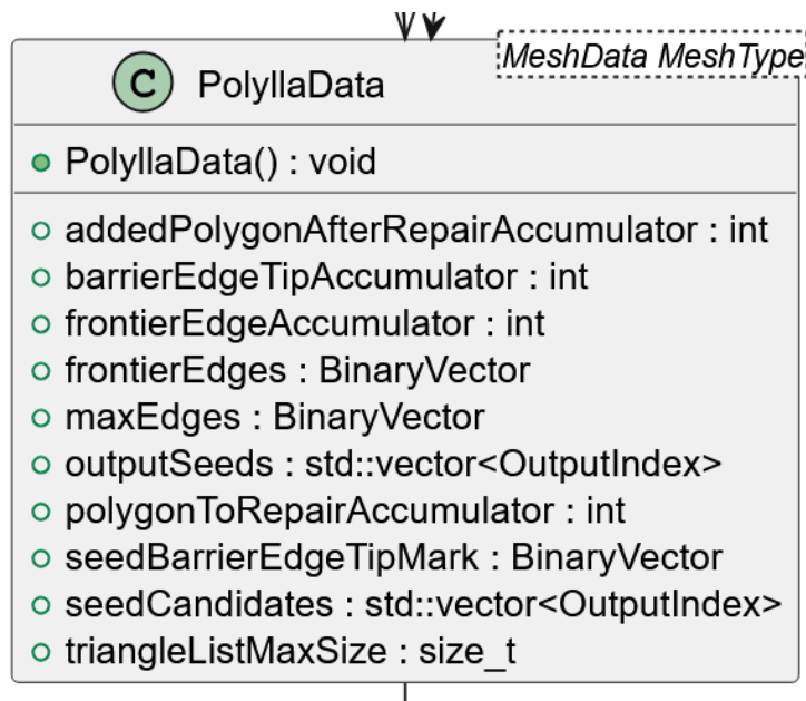
Figura 35: Representación UML de la clase PolyllaData
