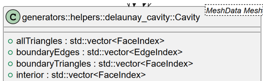
Figura 38: Representación UML de la estructura Cavity
