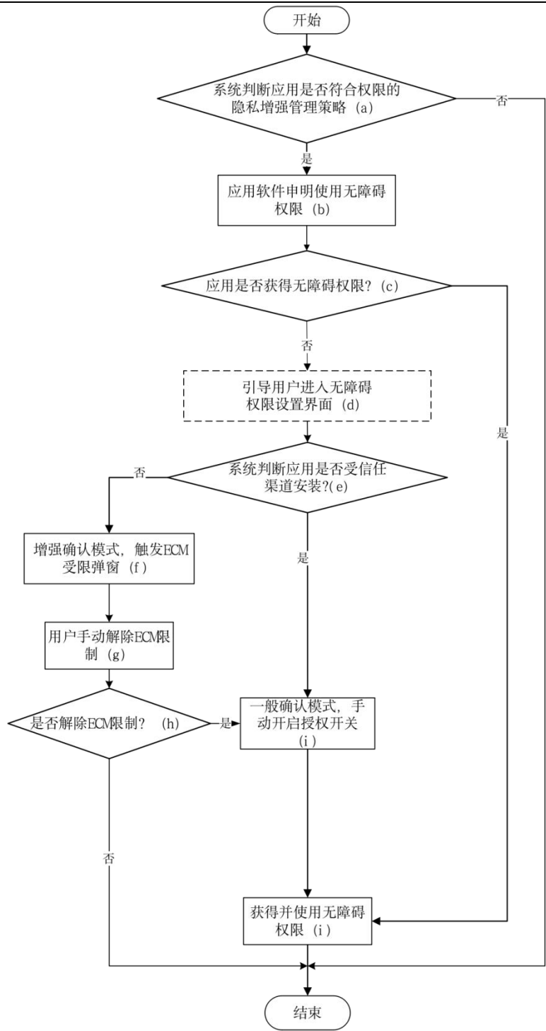
图 1 无障碍权限申请步骤
