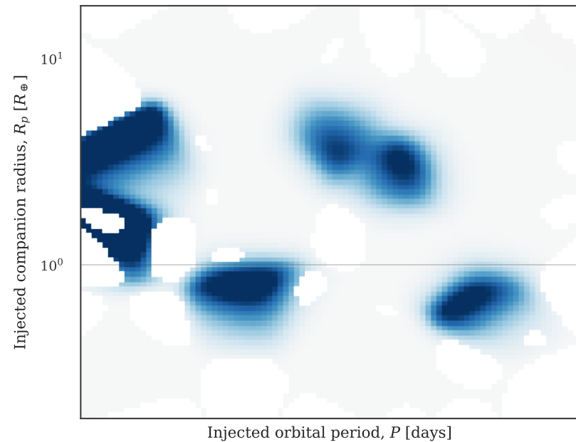
Tmag &lt; 17
