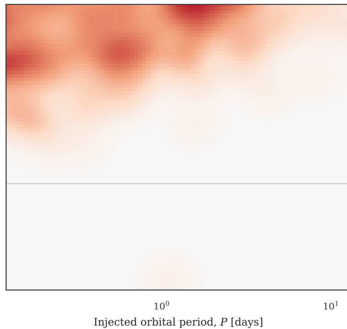
Tmag &gt;= 19
