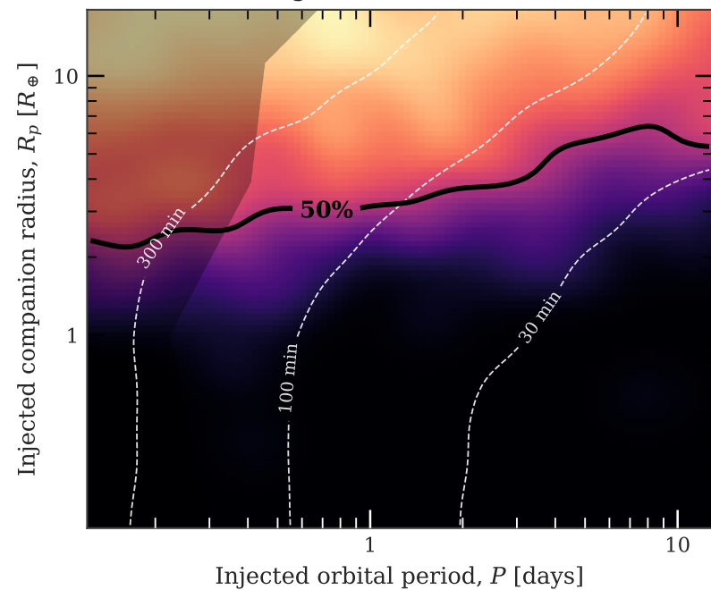
18 &lt;= Tmag &lt; 19: 696/2124 recovered
