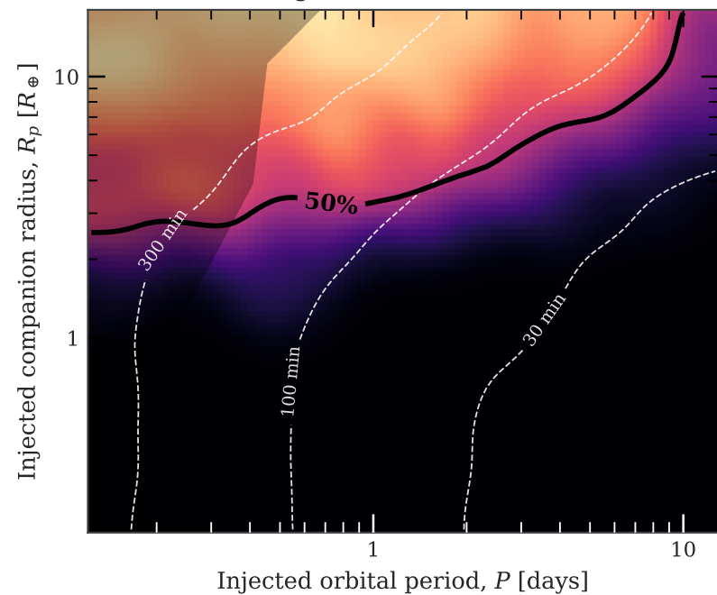
18 &lt;= Tmag &lt; 19: 589/2124 recovered
