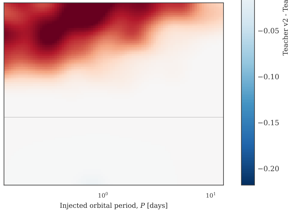
T_{\text{mag}} \geq 19
