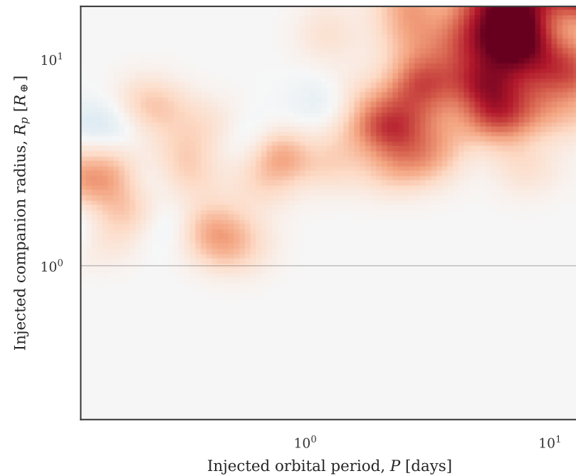
18 \leq T_{\text{mag}} < 19
