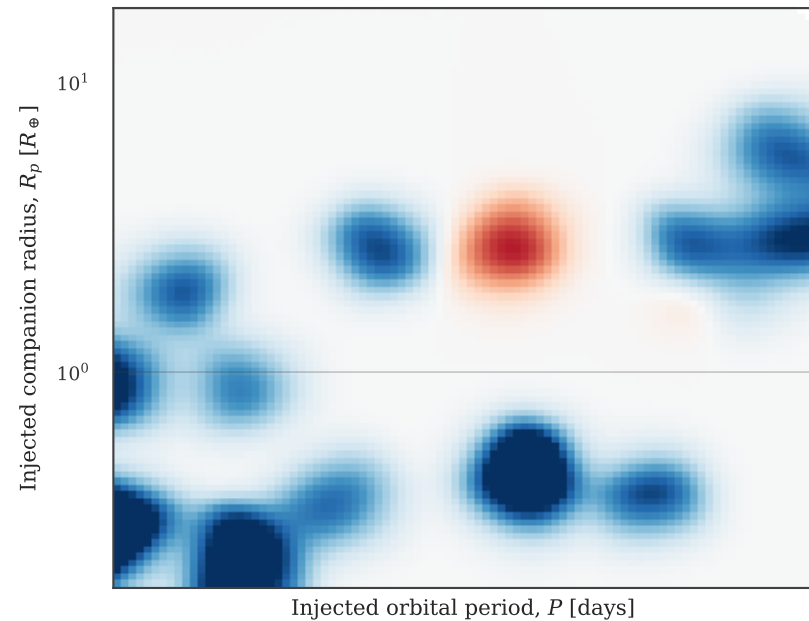
T_{\text{mag}} < 17
