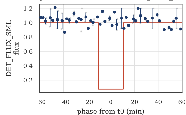
odd/even transit fold (EB check) odd_med=nan (n=0) even_med=0.322 (n=56) Δ=nan
