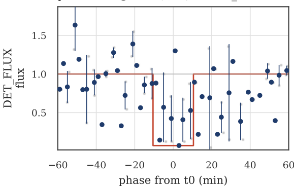
odd/even transit fold (EB check) odd_med=nan (n=0) even_med=0.322 (n=56) Δ=nan
