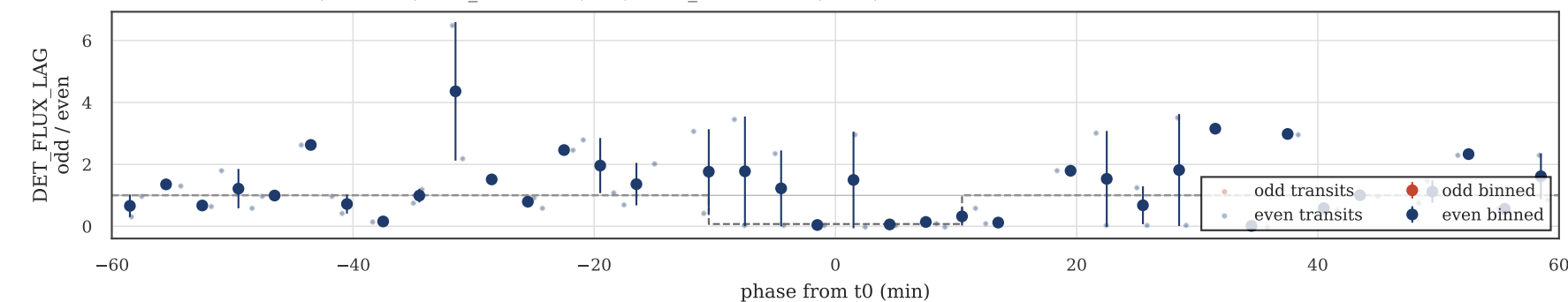
odd/even transit fold (EB check) odd_med=nan (n=0) even_med=0.322 (n=56) Δ=nan
