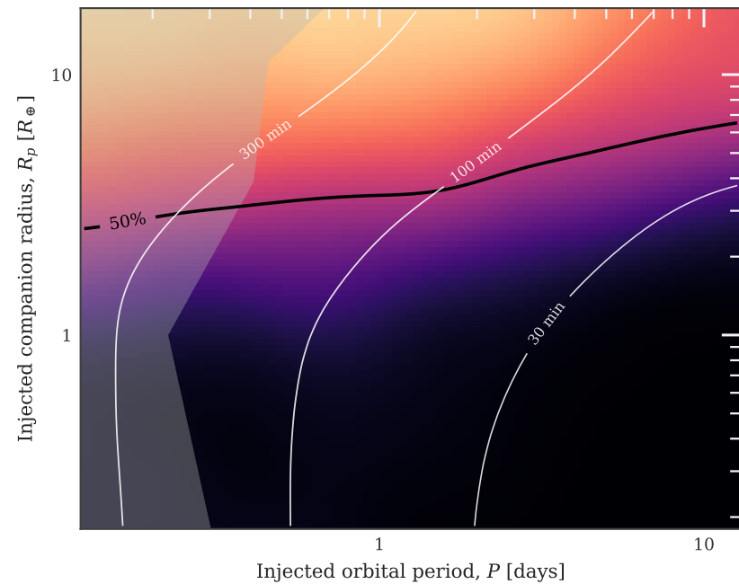
18 &lt;= Tmag &lt; 19: 1625/5026 recovered
