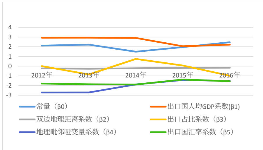
图8 影响因素的回归系数波动
