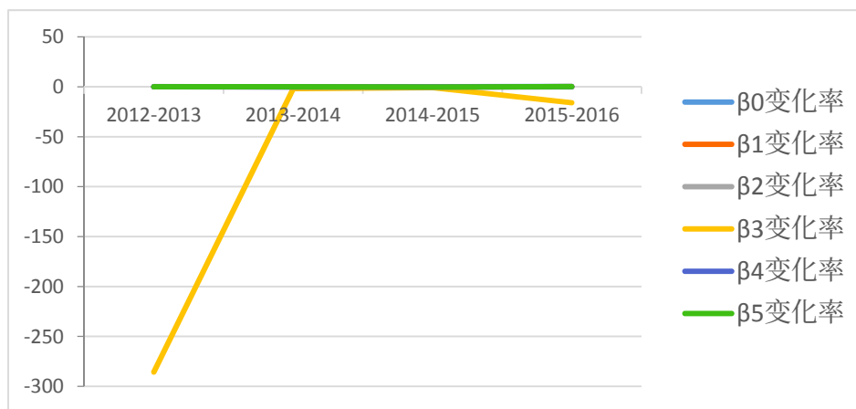
图9 邻年系数变化率
