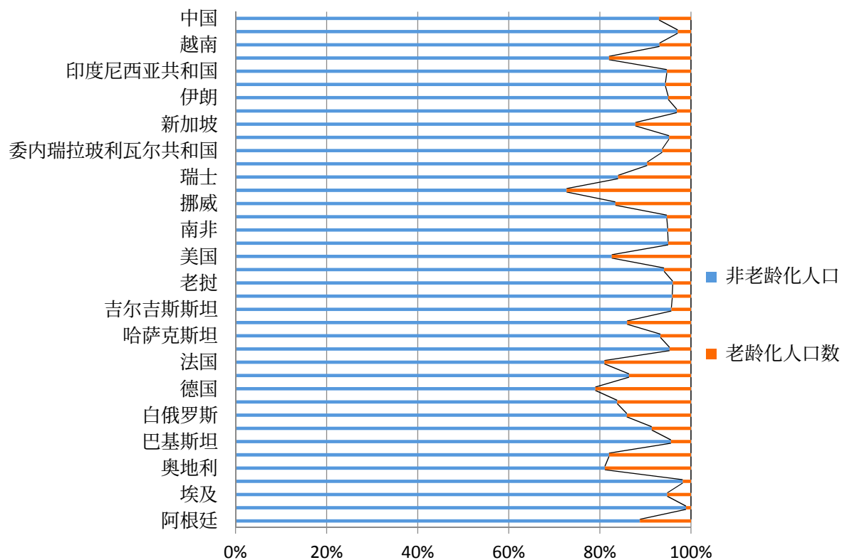
图 7 “一带一路”沿线国老龄化结构
