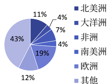
图 5 出口国所在洲分布
