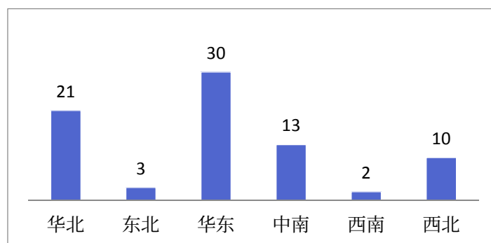
图 6 企业所在地分布
