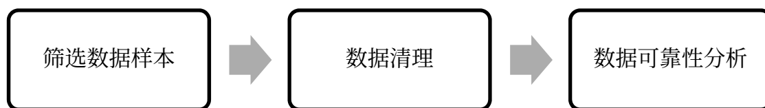
图 1 数据预处理过程
