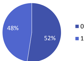
图 4 地理毗邻哑变量数量统计
