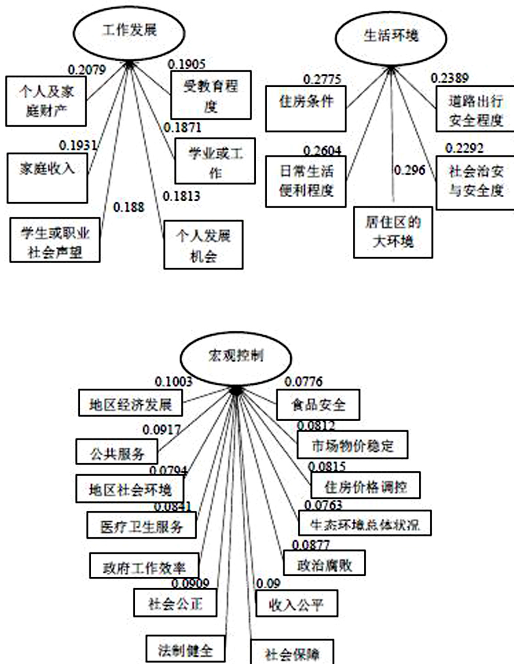
图 5 偏最小二乘 (pls-pm)权重系数图
