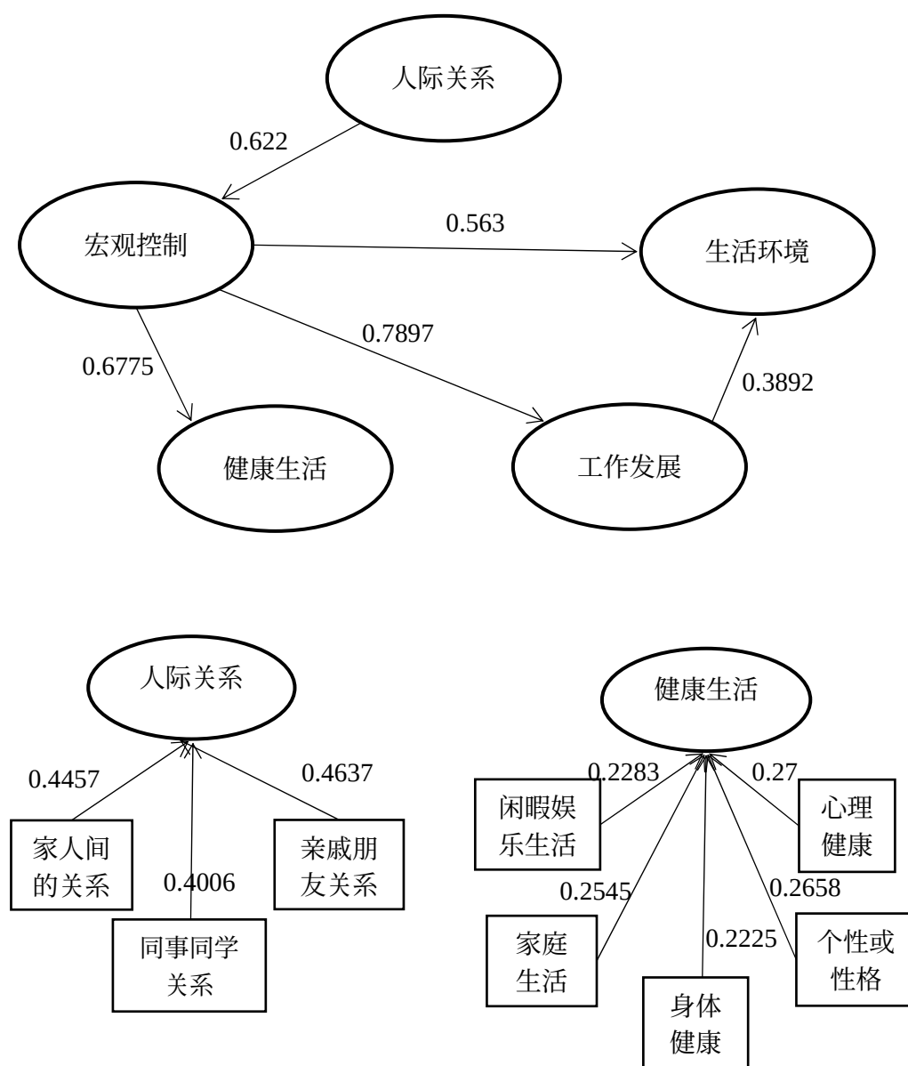
图 4 偏最小二乘 (pls-pm)路径图
