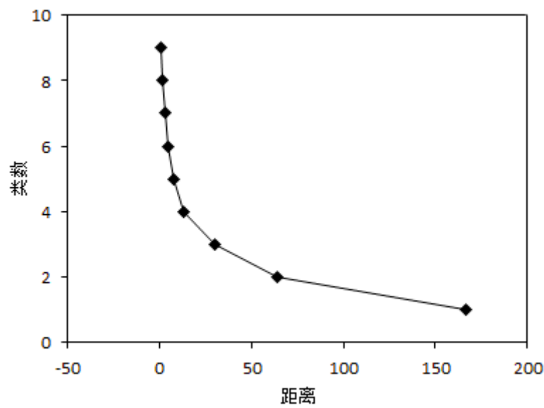
图 2 十大省市系统聚类分析碎石图
