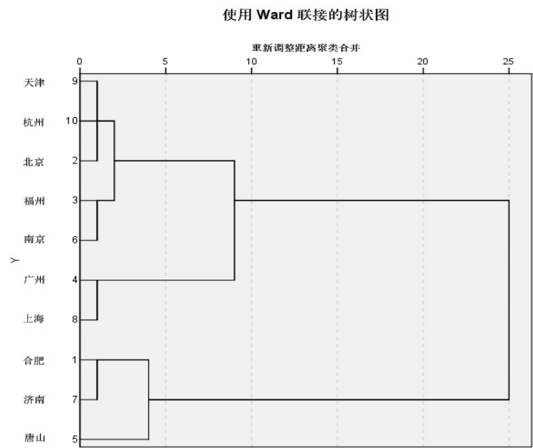
图 1 十大省市女性农民工压力状况的系统聚类树形图
