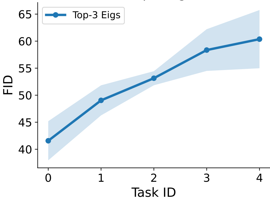
CIFAR10 - Top 3 Eigenvalues
