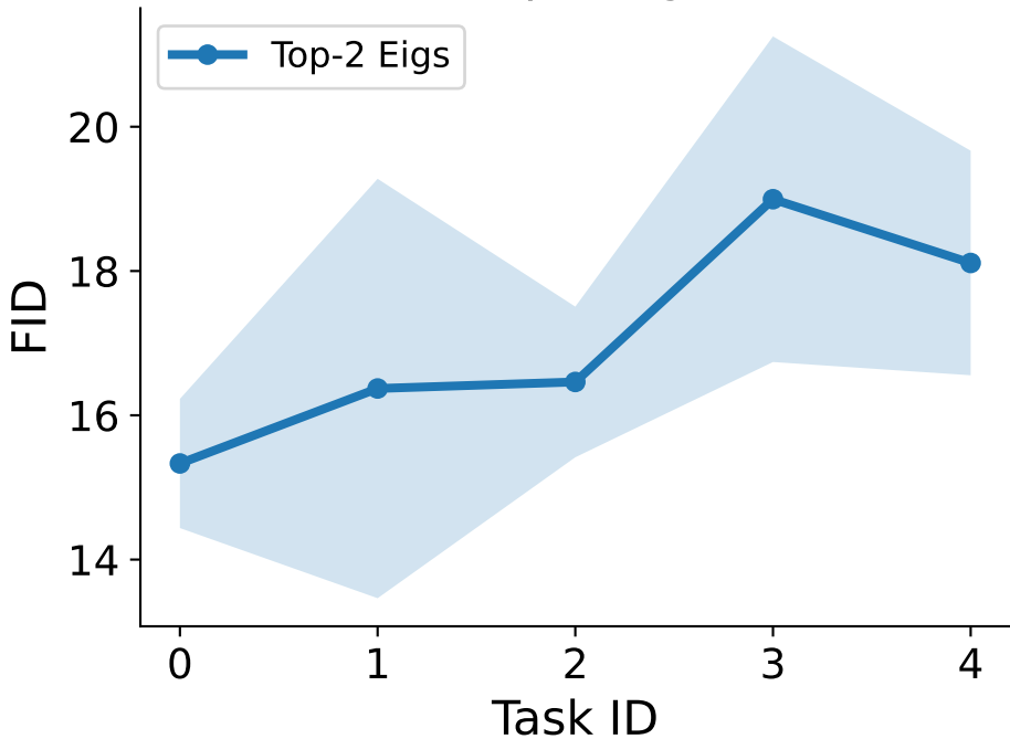
FMNIST - Top 2 Eigenvalues
