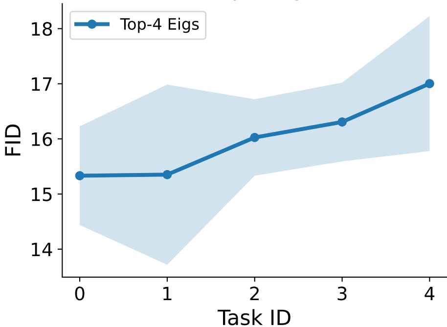
FMNIST - Top 4 Eigenvalues
