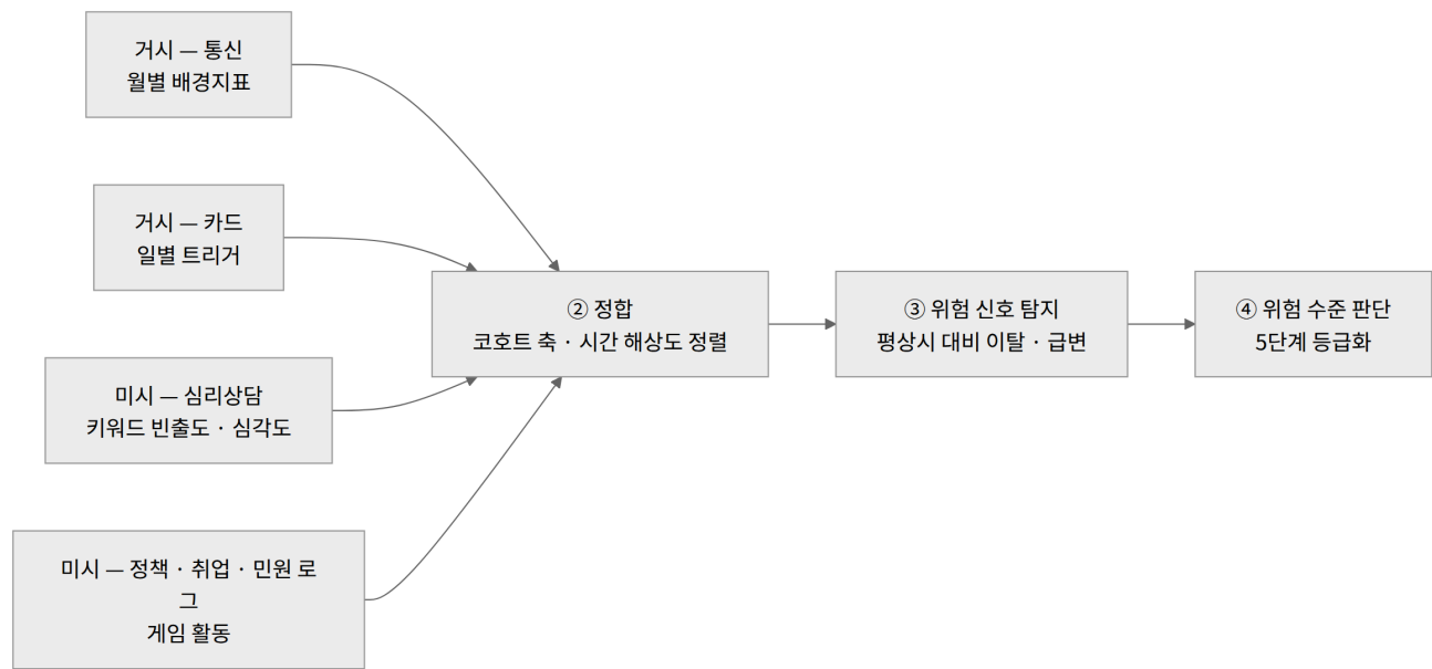
그림 3. 위험 탐지 에이전트 — ① 수집과 ②~④ 정합·탐지·판단
