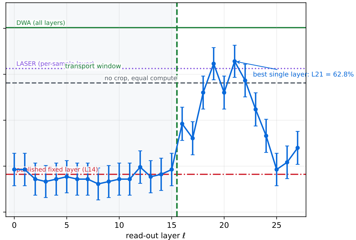
Qwen2-VL-7B, n=191
