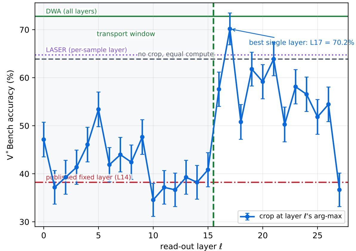
Qwen3-VL-2B, n=191
