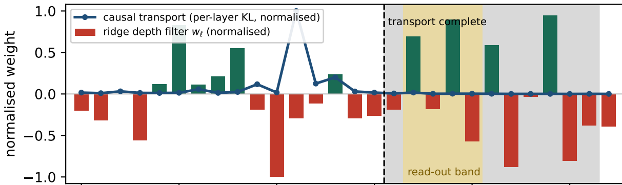
Qwen3-VL-2B
