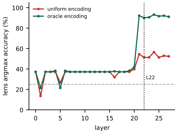
Qwen3-VL-2B
