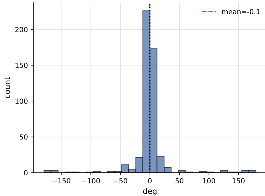
Longitude error (pred – truth)
