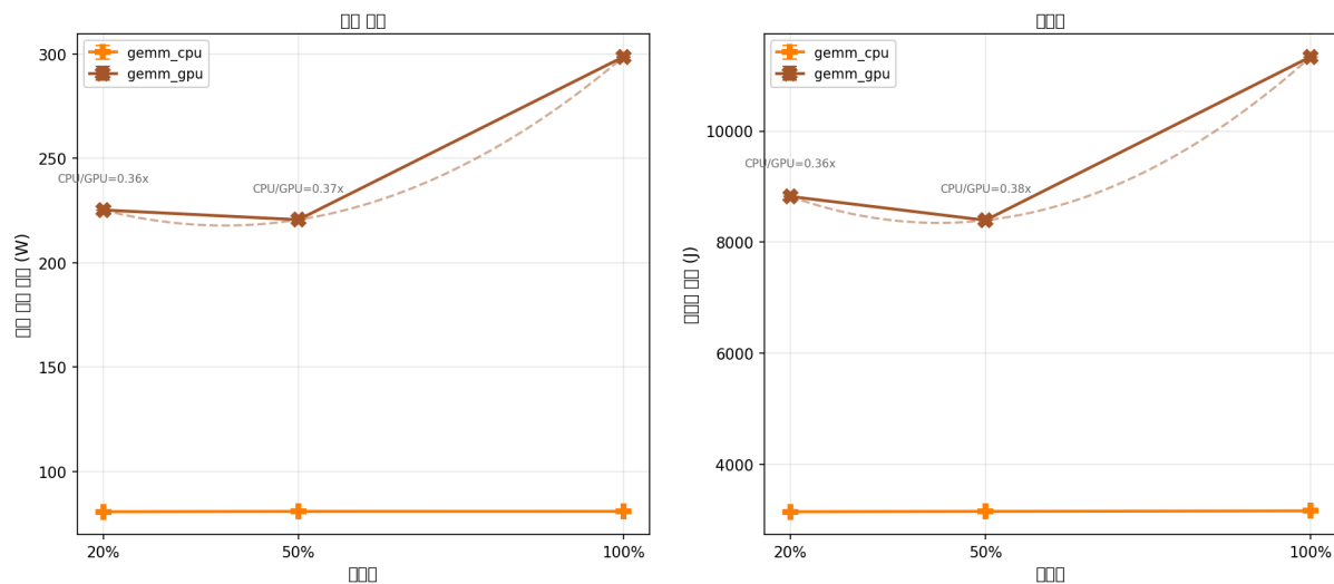
【그래프 5】 GEMM CPU vs GPU 전력 및 에너지 비교
