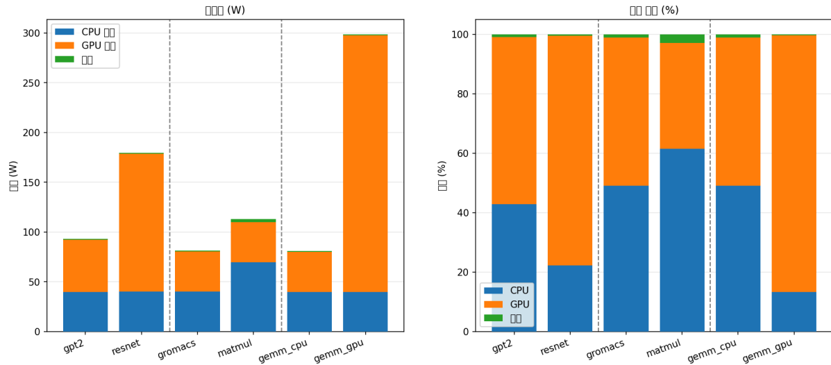
【그래프 4】 워크로드별 전력 분포 (100% 부하 기준)
