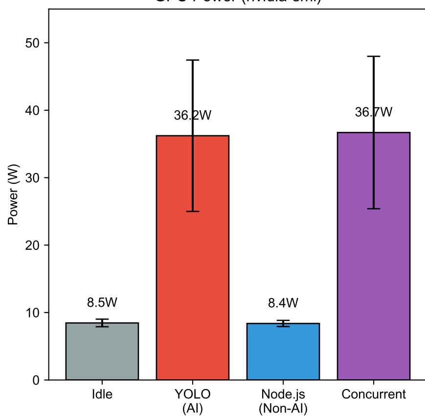
GPU Power (nvidia-smi)
