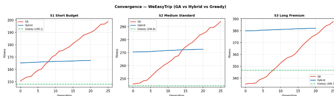
รูปที่ 4.1 กราฟ Convergence ของ GA และ Hybrid Algorithm ทั้ง 3 Scenarios
