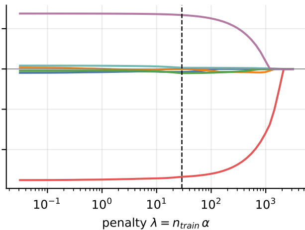
Lasso - ScalaTion
