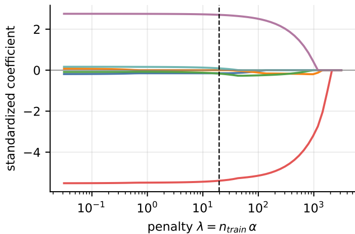
Lasso - statsmodels
