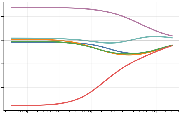
Lasso - ScalaTion
