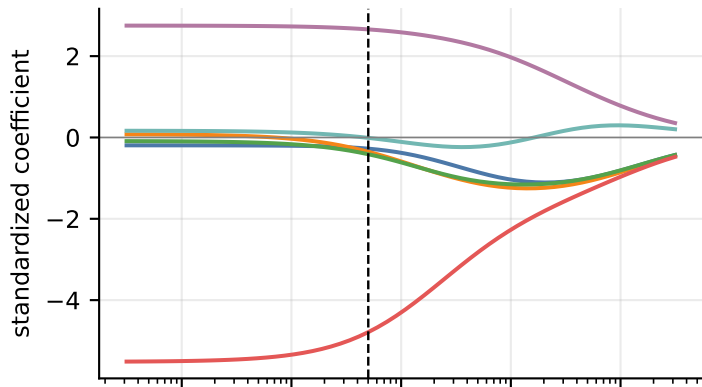
Lasso - statsmodels
