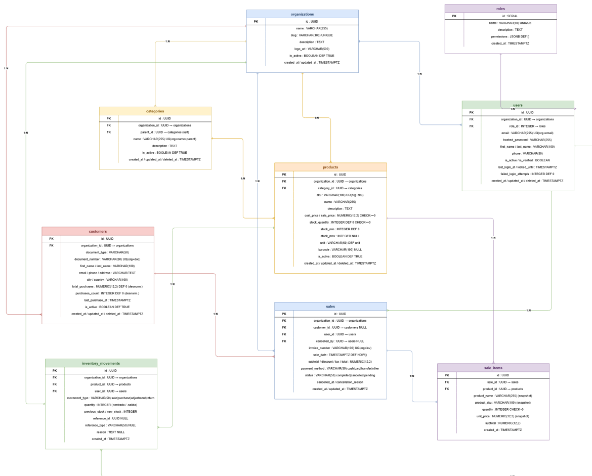
Figura 3.2: Diagrama Entidad-Relación
