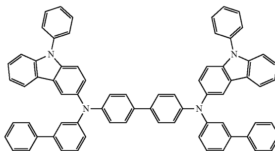
CP5
