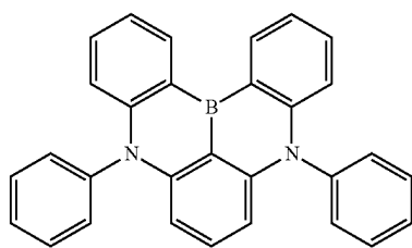
(DABNA-1)
