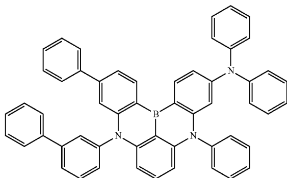
(DABNA-2)
