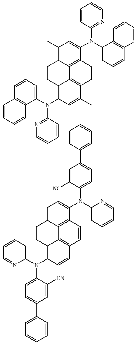
FD3
