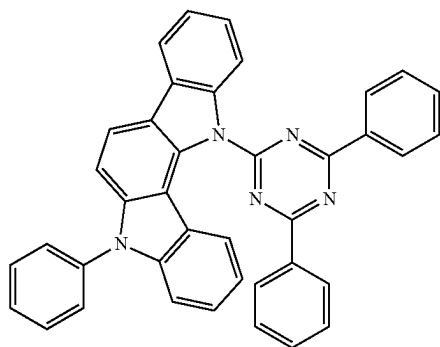
(PIC-TRZ2)
