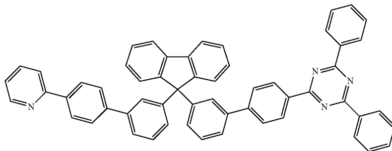
cpd 4
