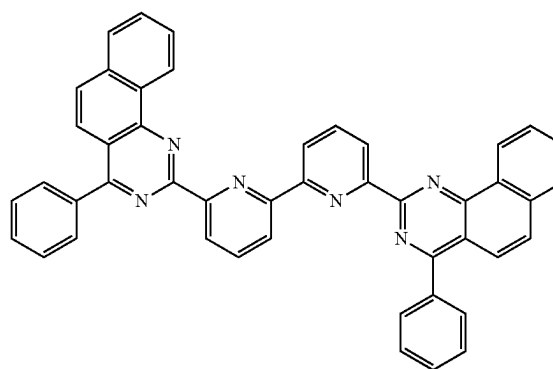
6,6'(P-Bqn)2BPy
