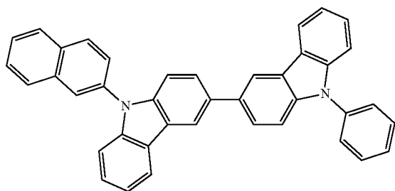
β NCCP
