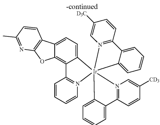
Ir(5mppy-d 3 ) 2 (mbfpypy-d 3 )
