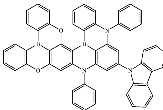
DF14
