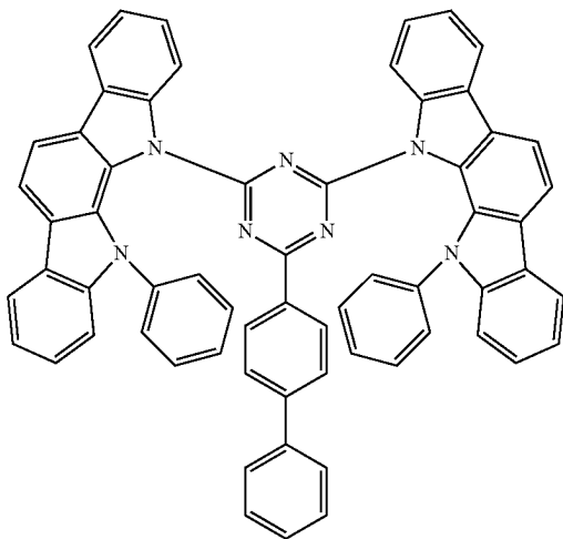
DF6(PIC-TRZ2)
