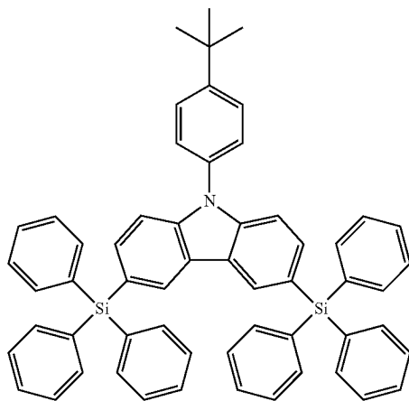
CzSi
