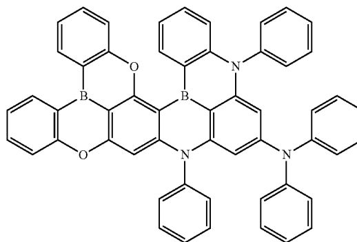
DFD13
