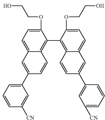
CN-BNA 6,6'-di-(3-cyanophenyl)-2,2'-bis-(2- hydroxyethoxy)-1,1'-binaphthalene
