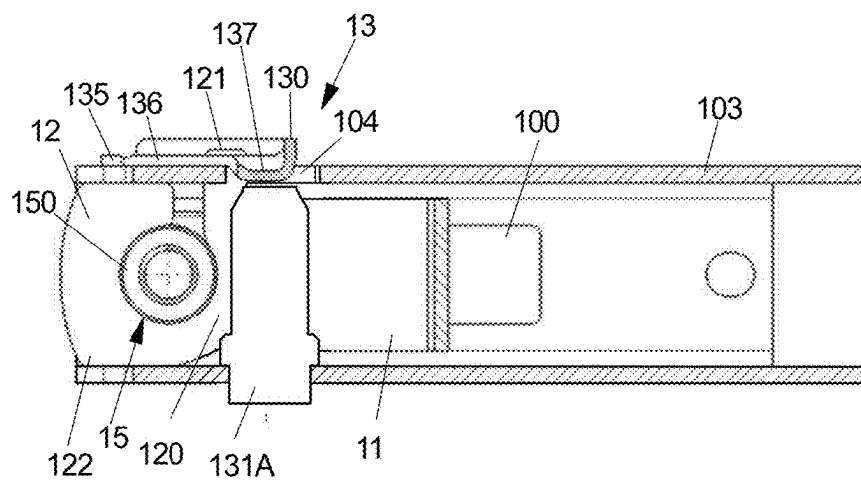
FIG. 3A (A-A)
