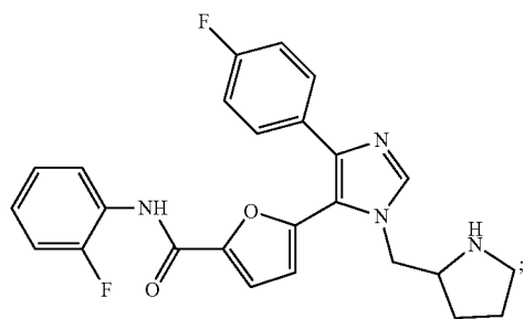
N-(2-fluorophenyl)-5-(4-(4-fluorophenyl)-1-(pyrrolidin-2-ylmethyl)-1H-imidazol-5-yl)furan-2-carboxamide
