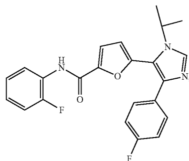
N-(2-fluorophenyl)-5-(4-(4-fluorophenyl)-1-isopropyl-1H-imidazol-5-yl)furan-2-carboxamide
