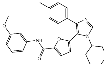
5-(1-cyclohexyl-4-(p-tolyl)-1H-imidazol-5-yl)-N-(3-methoxyphenyl)furan-2-carboxamide
