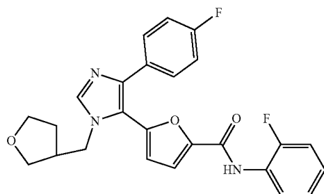
N-(2-fluorophenyl)-5-(4-(4-fluorophenyl)-1-((tetrahydrofuran-3-yl)methyl)-1H-imidazol-5-yl)furan-2-carboxamide
