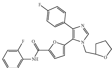
N-(2-fluorophenyl)-5-(4-(4-fluorophenyl)-1-((tetrahydrofuran-2-yl)methyl)-1H-imidazol-5-yl)furan-2-carboxamide
