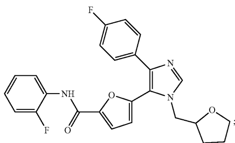
N-(2-fluorophenyl)-5-(4-(4-fluorophenyl)-1-((tetrahydrofuran-2-yl)methyl)-1H-imidazol-5-yl)furan-2-carboxamide
