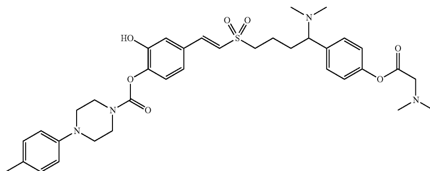
Compound P1-1-a
