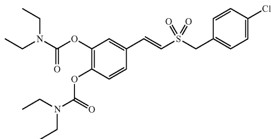
Compound D1-1
