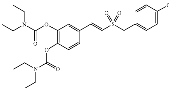
Compound D1-1
