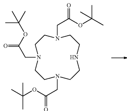
DO3A(tertBuO) 3
