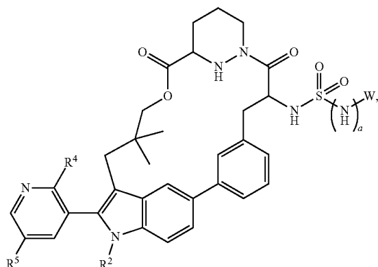
Formula VIa-3
