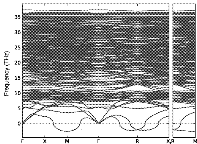
Type-I \text{Ca}_8\text{C}_{46} phonon dispersions
