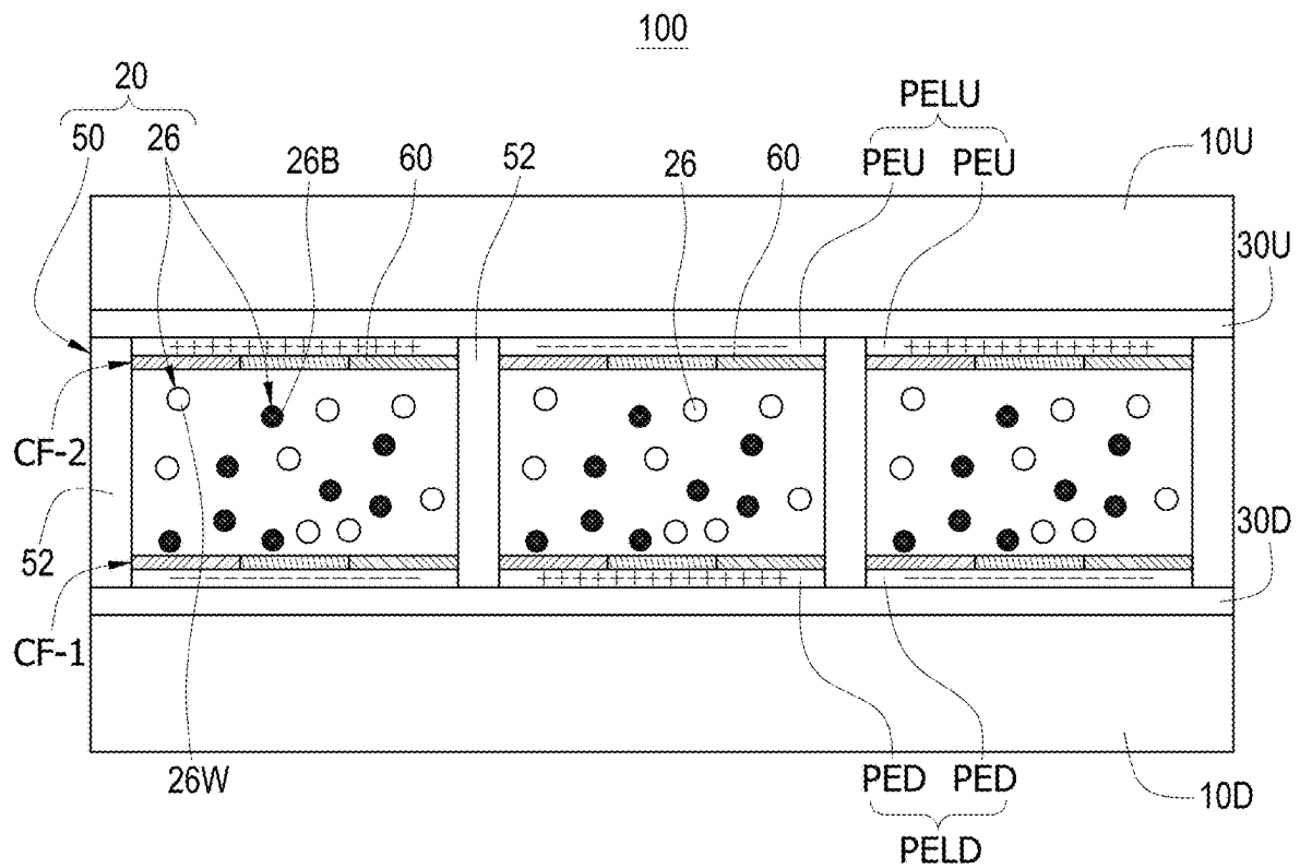
FIG.20C
