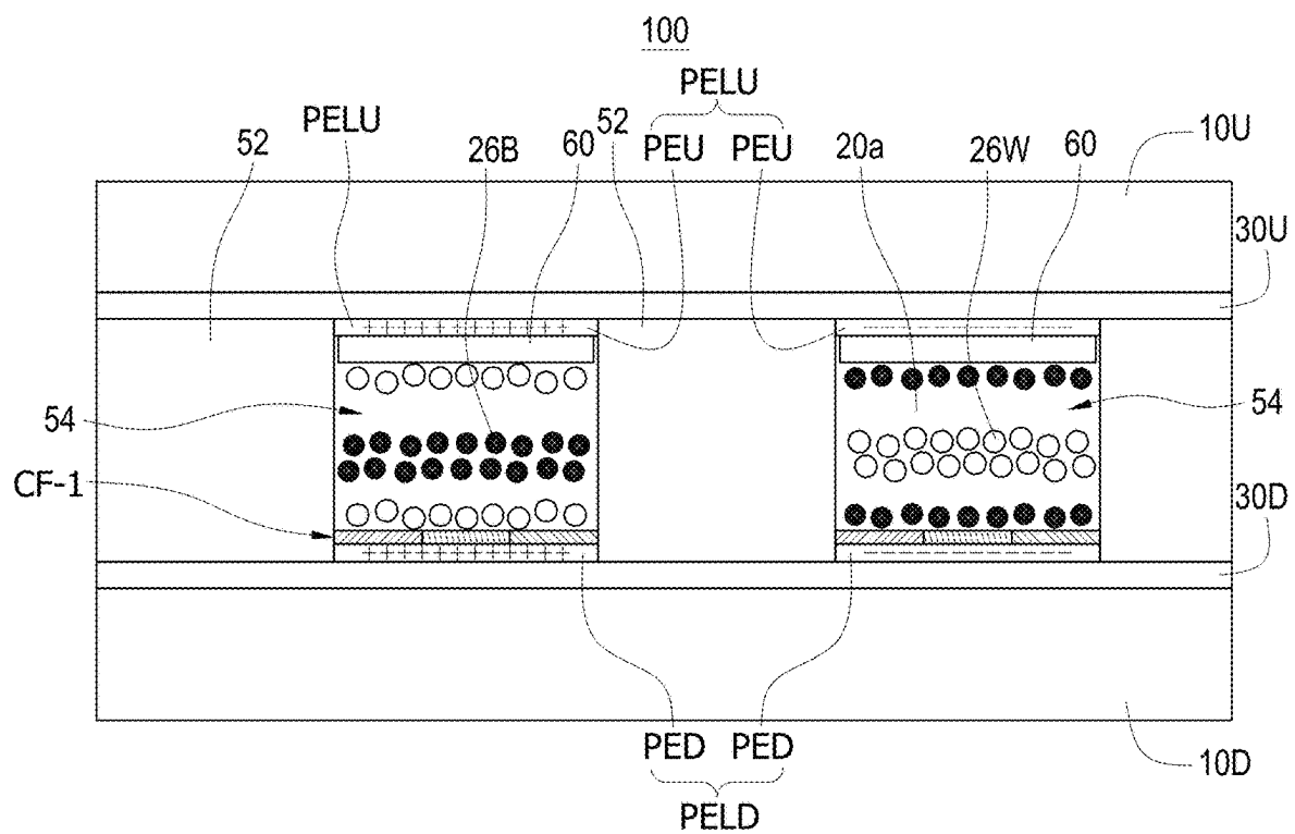
FIG. 16D
