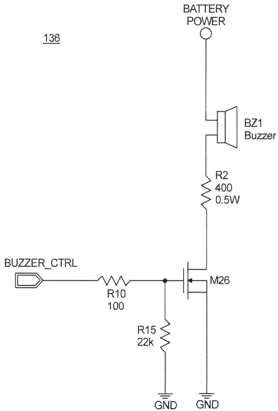
Buzzer Module
